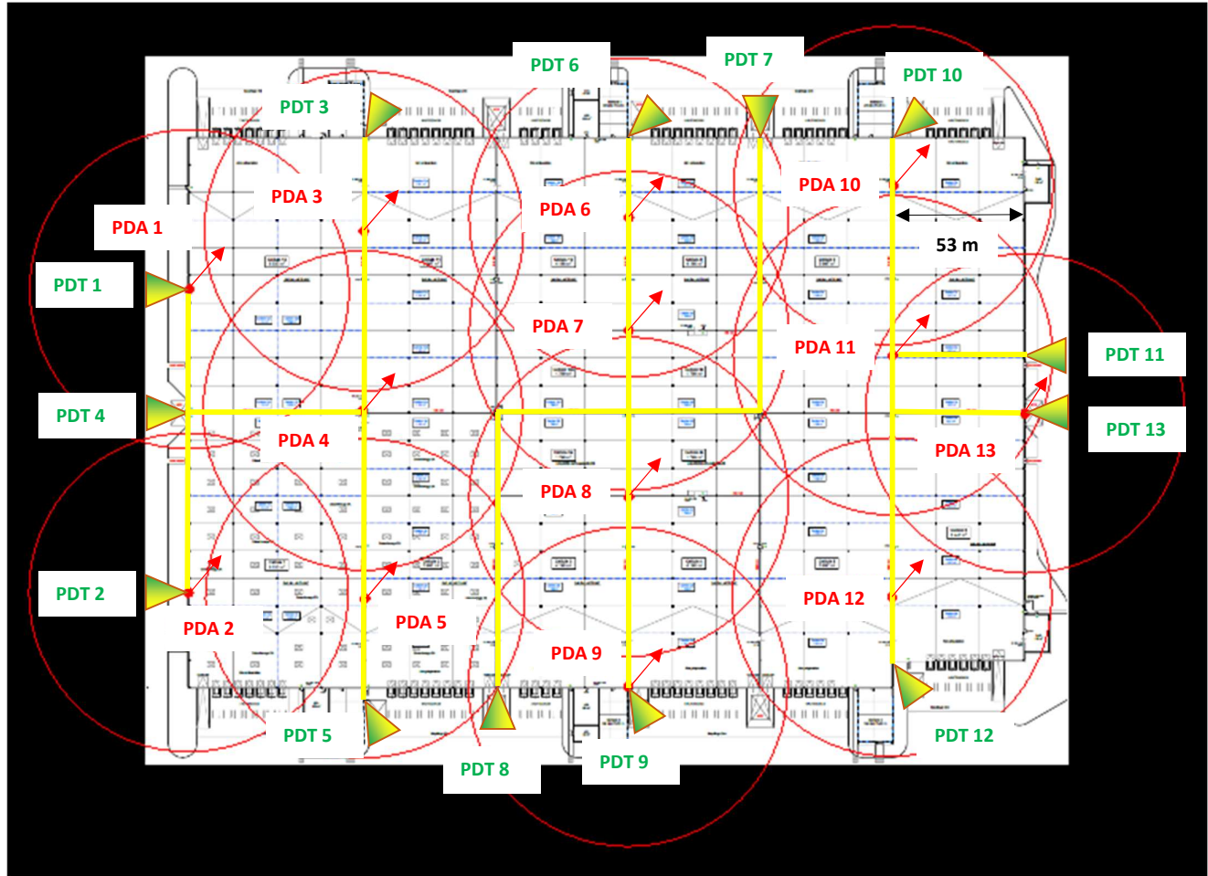
Implantation des paratonnerres, conducteurs de descente et prises de terre.
